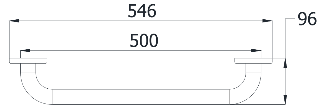
VISTA SUPERIOR
