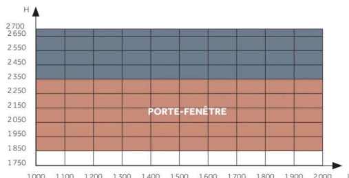
FRANÇAISE SERRURE - 2 vantaux
