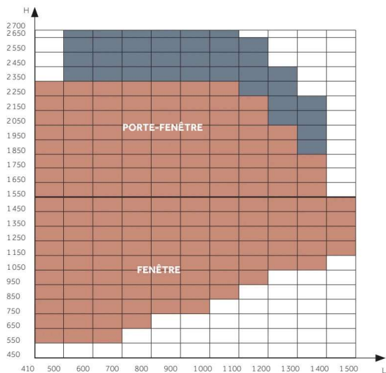
OSCILLO-BATTANT - 1 vantail
