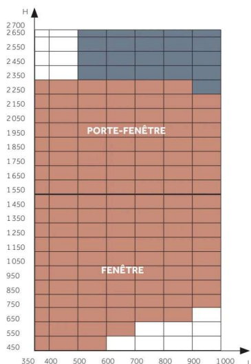
FRANÇAISE - 1 vantail
