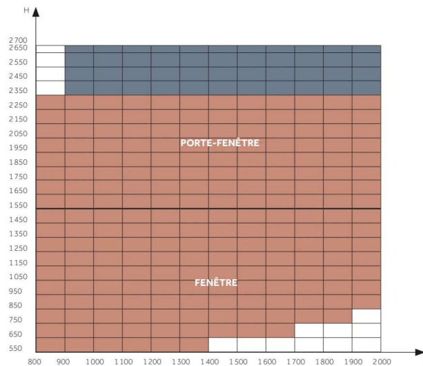
OSCILLO-BATTANT - 2 vantaux
