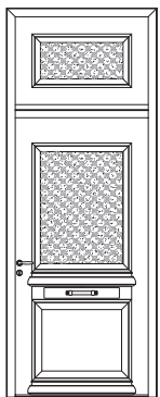
Athéna avec imposte coordonnée. H 3050 / L 1105.
