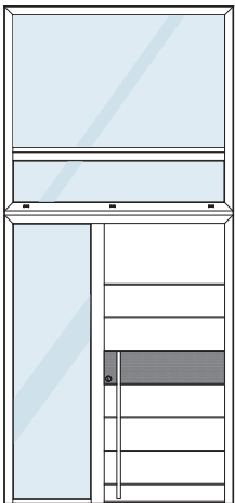
Oxygène avec fixe en dormant et imposte vitrée avec traverse et assemblage adaptés aux dimensions. H 3900 / L 1726.
