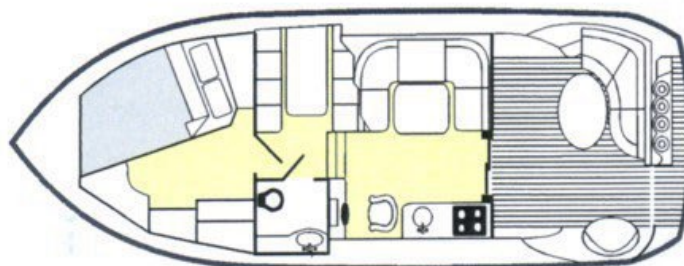
sedan 34 dinette
