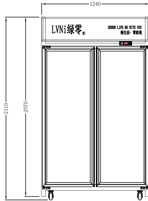
ELEVATION (前视)
