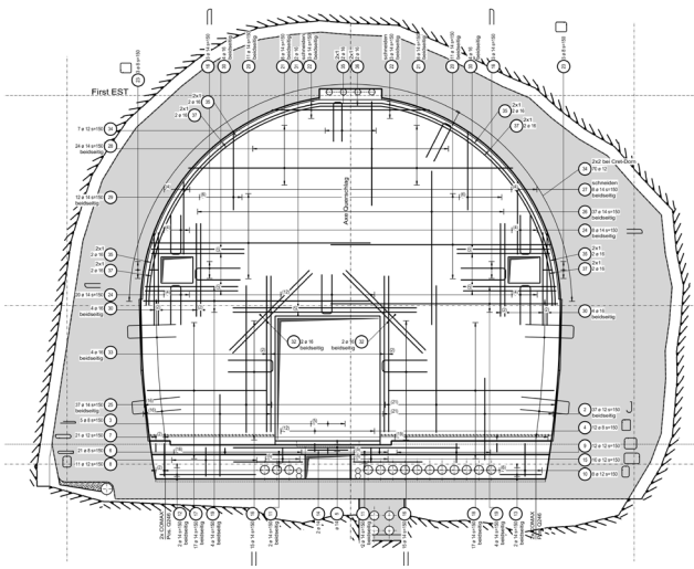
Querschnitt Einspurtunnel Amsteg Ost, Bewehrung (BIM Software Allplan)
