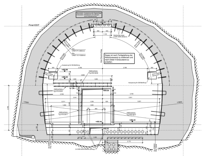
Querschnitt Einspurtunnel Amsteg Ost, Schalung (BIM Software Allplan)
