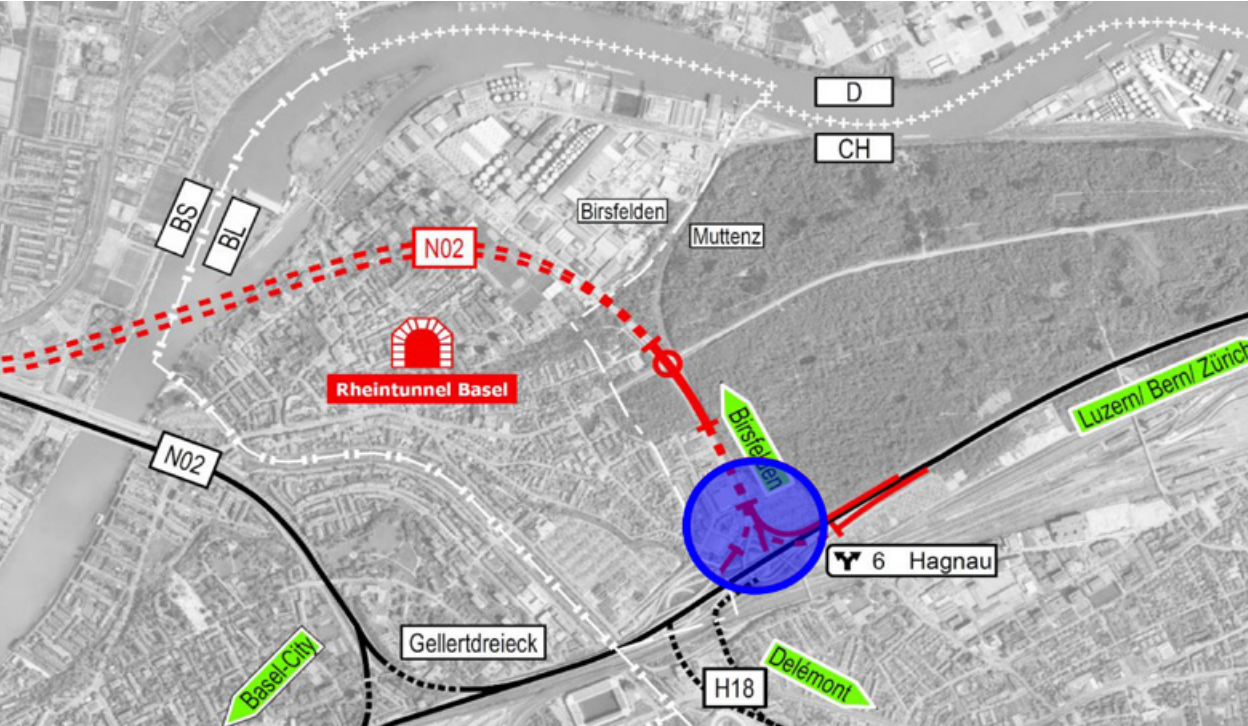
Situation Rheintunnel Basel, Überführung der Hafенbahn an der Verzweigung Hagnau (blauer Kreis)
