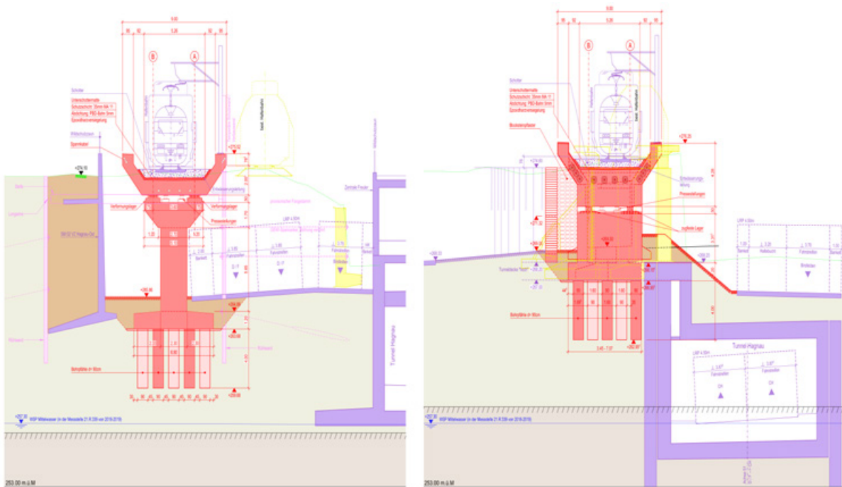
Querschnitt 2 (Achse 30) und Querschnitt 3 (Achse 10)
