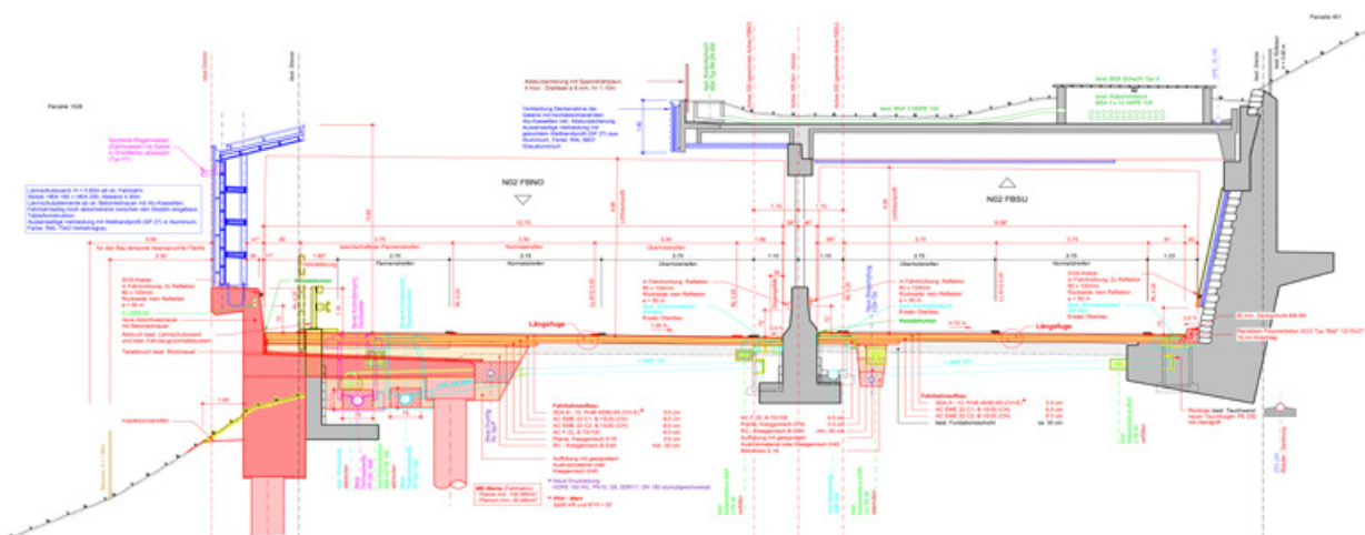
Querschnitt Stützkonstruktion auf Ortbetonbohrpfählen mit Lärmschutzwand
