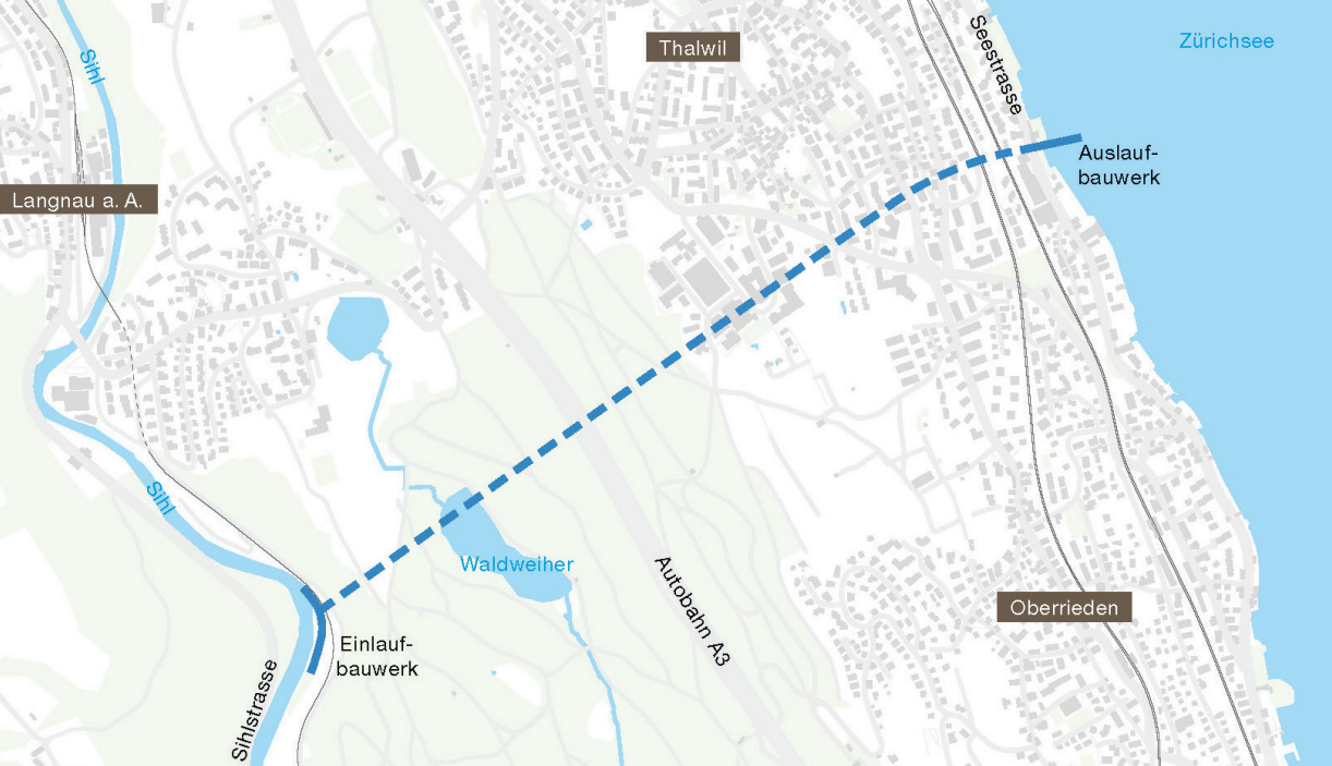
Situation Entlastungsstollen Thalwil
