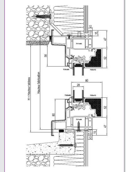
Isolation intérieure de 100 mm (possible de 70 à 160 mm)
