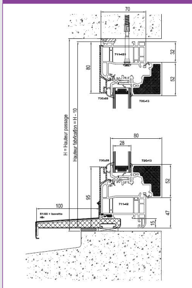
Pièce d'appui de 100 mm en base
