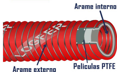
Mangueira PTFE tipo III - 3 películas
