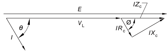
(d) \cos \theta = \cos \phi (maximum voltage drop condition)
