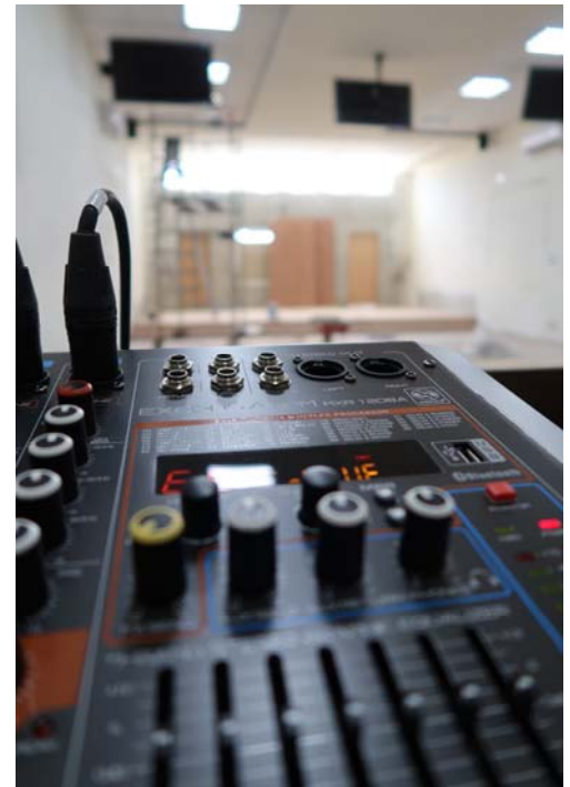
Instalasi sistem audio GECKO pada Baptist Citong Church
