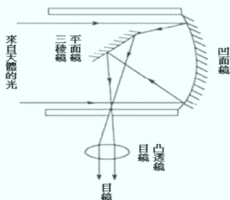
反射式天文望遠鏡的原理圖
