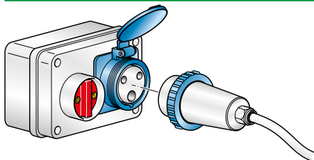
MCH-3/EM - 32A 2P+E plug not supplied MCH-3/EM - Spina 32A 2P+T non in dotazione
