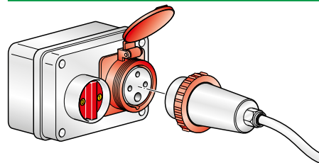
MCH-3/ET - 16A 3P+E plug not supplied MCH-3/ET - Spina 16A 3P+T non in dotazione
