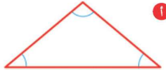
مُثلث
