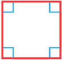
مُرَبَّع
