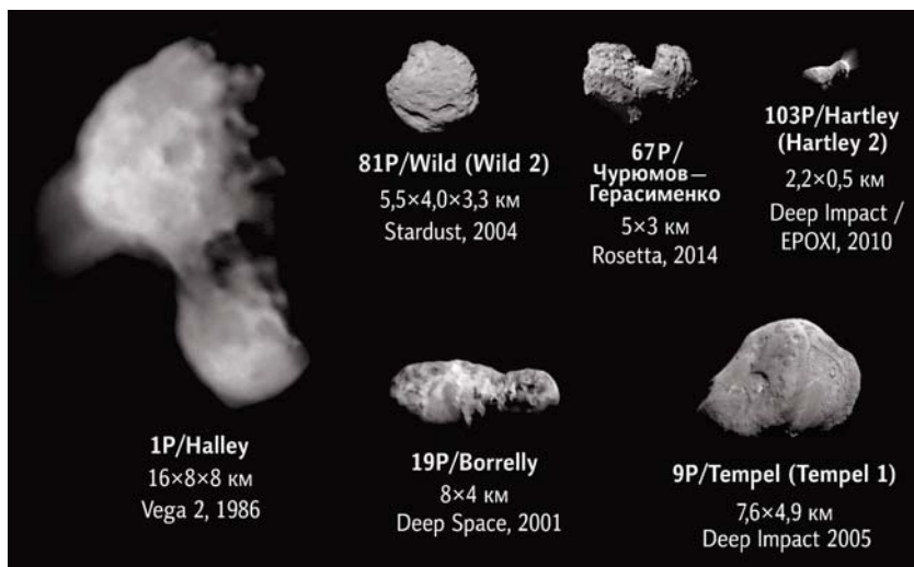
Рис. 7.21. Кометы, к которым осуществлялись миссии автоматических зондов. Фотографии ядер комет предоставлены РАН, NASA, ESA.
