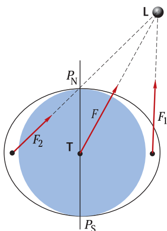
Рис. 8.26. Причина прецессии оси вращения планеты Т – в асимметрии сил, действующих со стороны небесного тела L на экваториальное «вздутие» планеты.
