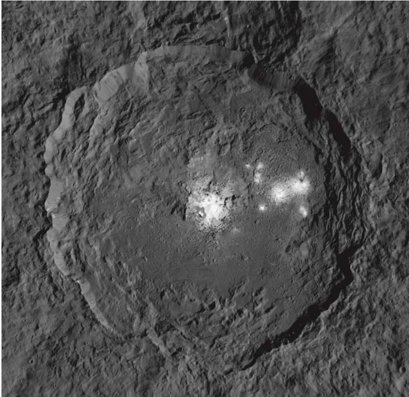
Рис. 7.2. Кратер Оккатор диаметром 80 км. На его дне видны отложения льда или солей. Это самое яркое из светлых пятен, замеченных «Хабблом».
