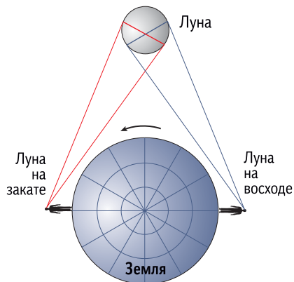
Рис. 1.9. Горизонтальный параллакс.
