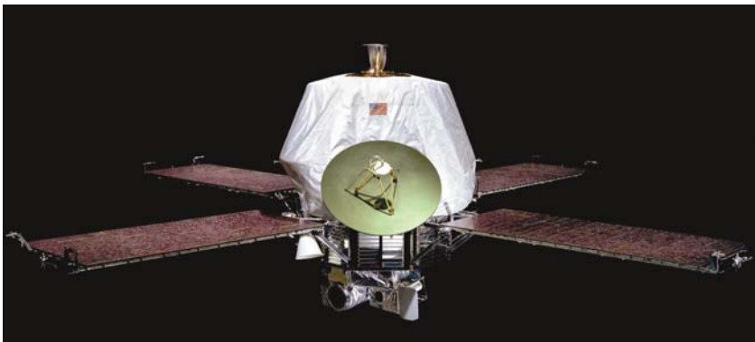
Рис. 5.1. «Маринер-9», первый искусственный спутник Марса (NASA).
