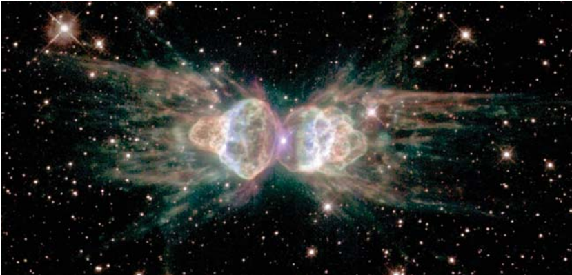
Рис. 12.22. Планетарная туманность «Муравей». Фото космического телескопа «Хаббл».
