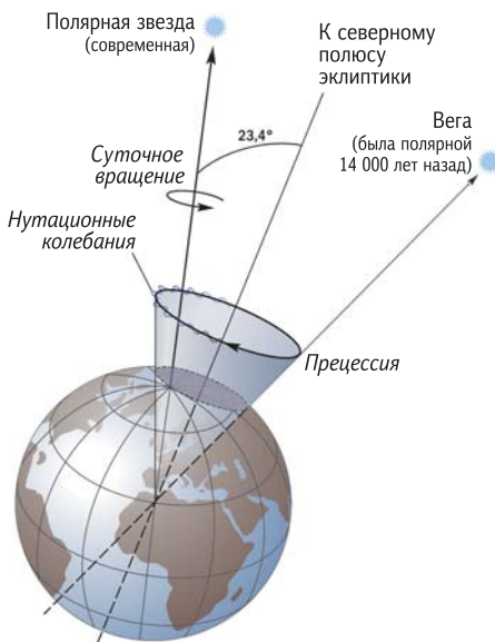
Рис. 8.28. Прецессия земной оси с мелкими нутационными колебаниями.
