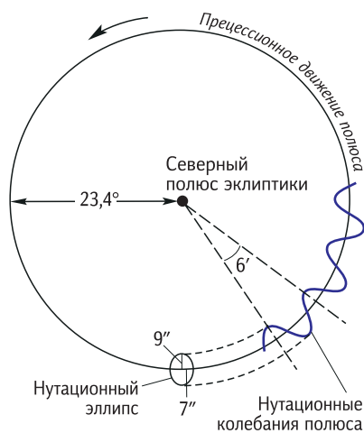
Рис. 8.31. Сложное движение земной оси можно представить как сумму прецессии и нутации.
