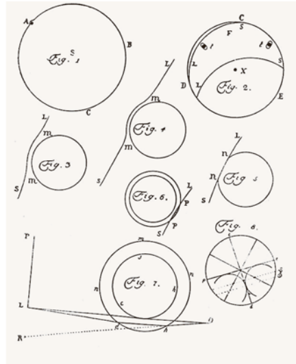
Рис. 1.32. М. В. Ломоносов наблюдает за прохождением Венеры по диску Солнца 26 мая 1761 г. из своей петербургской квартиры. Справа — иллюстрации Ломоносова в его рукописи «Явление Венеры на Солнце...» (1761).
