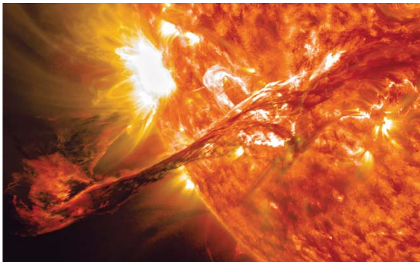
Рис. 10.19. Выброс протуберанца 3 февраля 2016 г. Фото: NASA.
