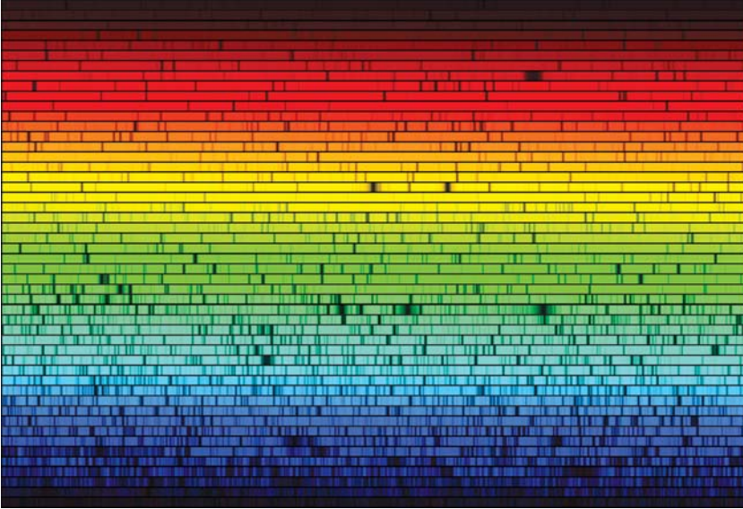
Рис. 11.6. Спектр Солнца или яркой звезды для детального исследования можно сильно растянуть, нарезать на кусочки и сложить стопкой от красного конца к синему. Технически это делается с помощью двух скрещенных дифракционных решеток: одна создает спектр с высокой дисперсией, соседние порядки которого частично накладываются друг на друга, а вторая раздвигает их в перпендикулярном направлении.
