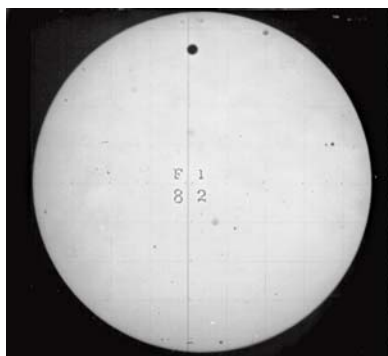
Рис. 1.34. Прохождение Венеры по диску Солнца. Слева — фото 6 декабря 1882 г., справа — 8 июня 2004 г.
