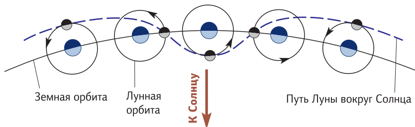
Рис. 3.32. Траектория Луны, как ее часто неверно изображают.
