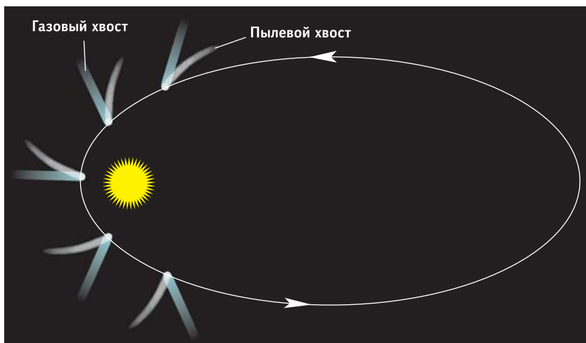
Рис. 7.20. Схема формирования хвостов кометы.
