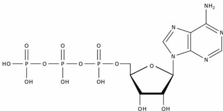
аденозинтрифосфат (АТФ)
