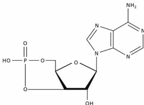
циклический аденозинмонофосфат (цАМФ)
