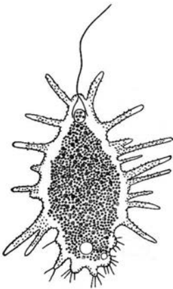
жгутиконосец мастигамеба
