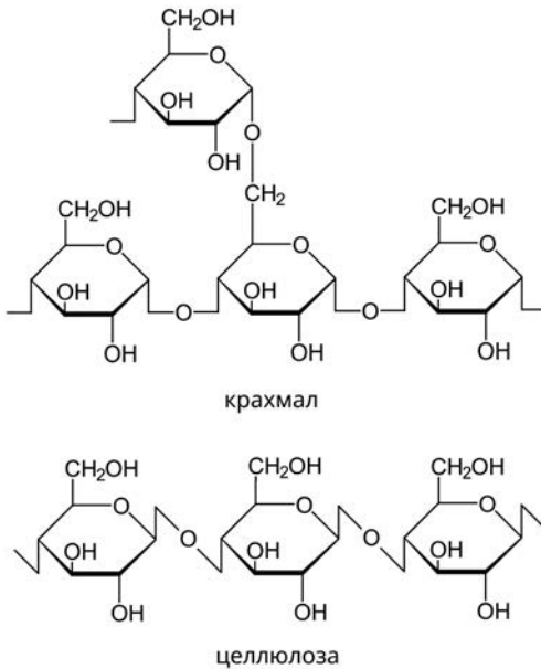
Рис. 6.4. Полисахариды: крахмал и целлюлоза
