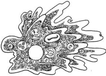
обыкновенная амеба
