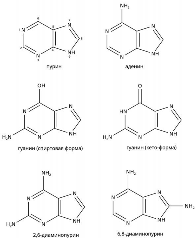
Рис. 7.2. Пуриновые азотистые основания
