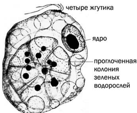
Рис. 10.5. Жгутиконосец Collodictyon
