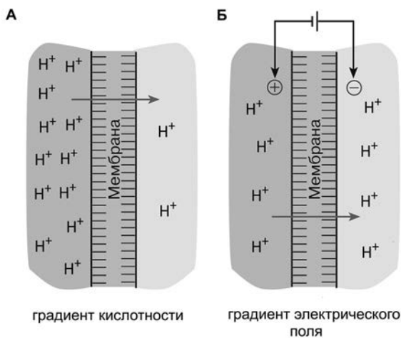
Рис. 11.2. Протонный потенциал. А — концентрационный потенциал, где протондвижущая сила создается просто за счет разности концентраций протонов. Б — электростатический потенциал: протоны стремятся по закону Кулона двигаться от “плюса” к “минусу”, даже если их концентрации всюду равны. В общем случае протонный потенциал имеет и концентрационную, и электростатическую составляющую
