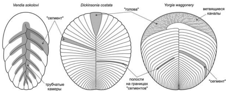
Рис. 16.5. Некоторые вендобионты
