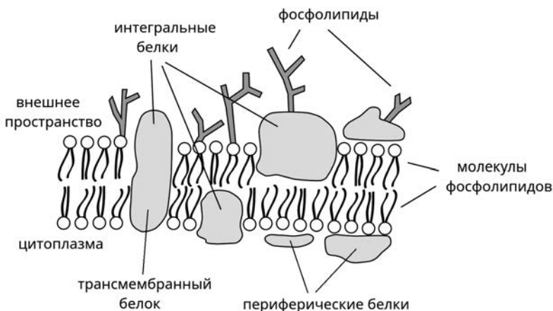
Рис. 5.4. Общая схема типичной клеточной мембраны
