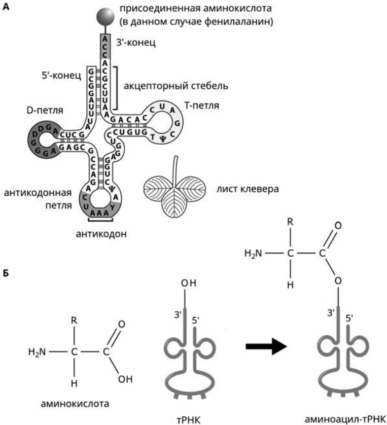
Рис. 9.5. Транспортная РНК. А – схема молекулы аминоацил-тРНК, Б – присоединение аминокислоты к тРНК
