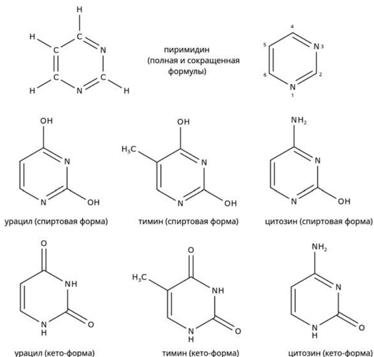
Рис. 7.1. Пиримидиновые азотистые основания
