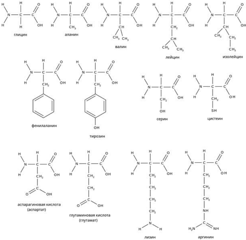
Рис. 3.3. Некоторые протеиногенные аминокислоты
