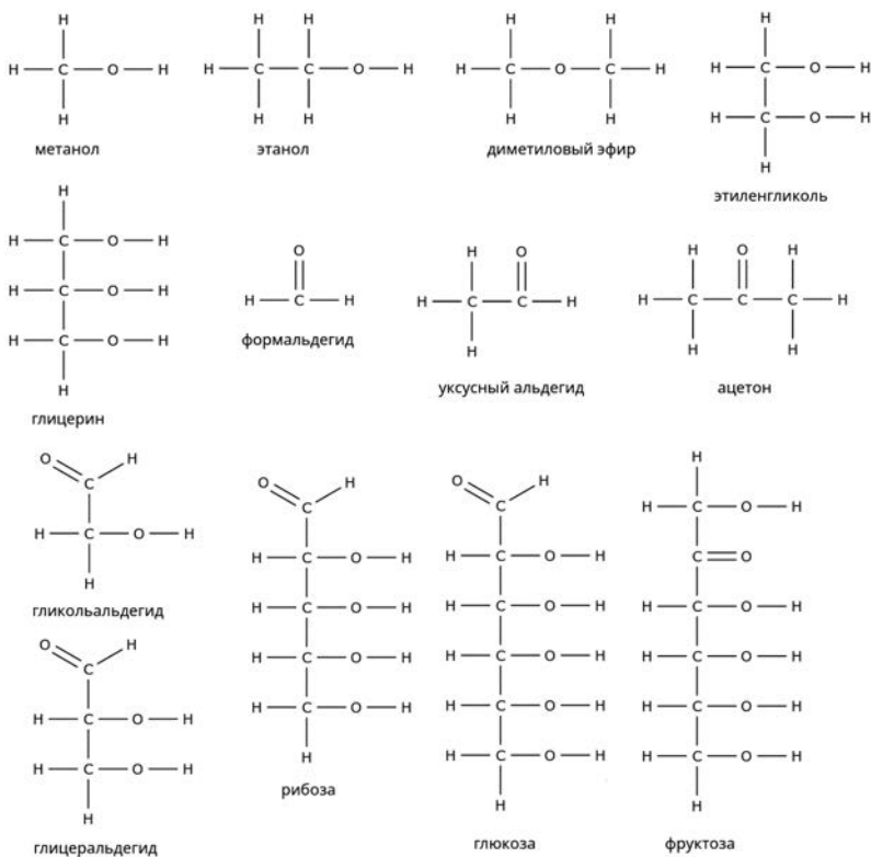
Рис. 1.6. Спирты, простые эфиры, альдегиды, кетоны, углеводы
