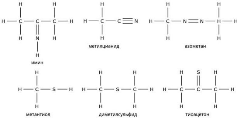
Рис. 1.9. Примеры бескислородных органических соединений
