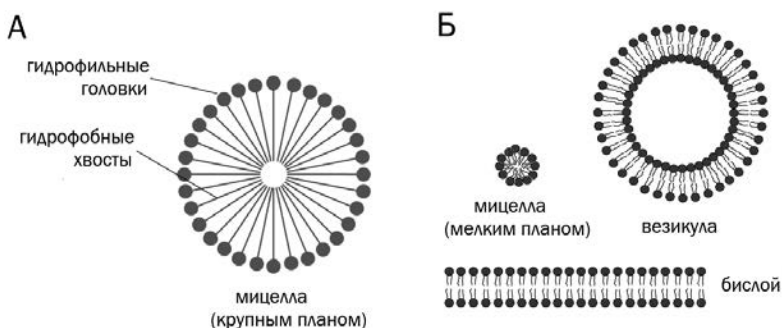
Рис. 5.3. Способы самоорганизации молекул липидов в растворе
