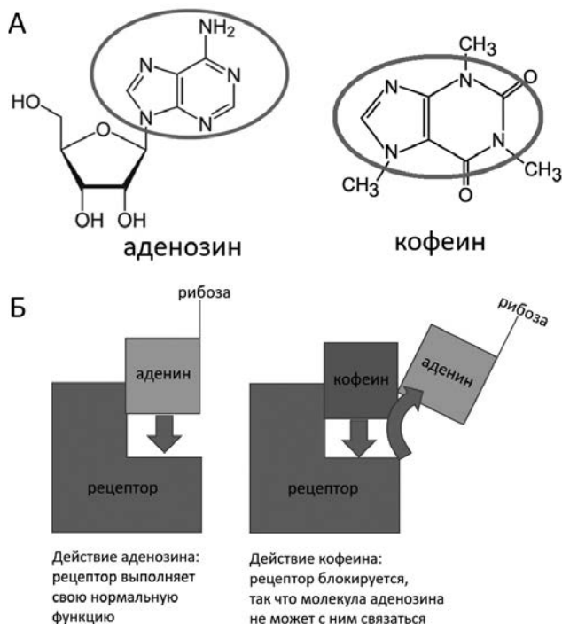
Рис. 7.4. Аденозин (А), кофеин (Б) и механизм действия кофеина на нервную систему (В). Пояснения в тексте
