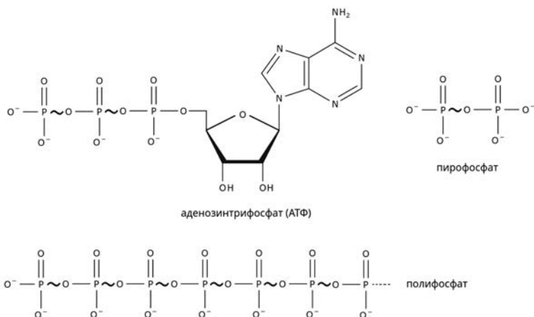
Рис. 11.1. Химические источники энергии
