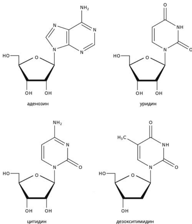
Рис. 7.3. Примеры нуклеозидов
