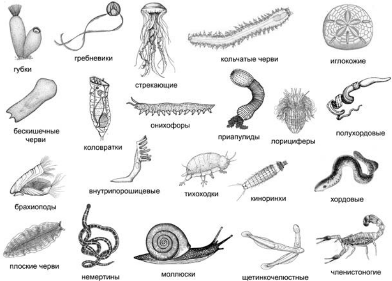
Рис. 15.11. Представители некоторых (далеко не всех) типов многоклеточных животных
