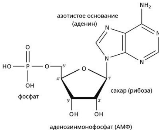
Рис. 7.5. Типичный нуклеотид
