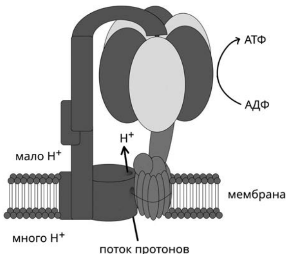
Рис. 11.3. Протонная АТФ-синтаза
