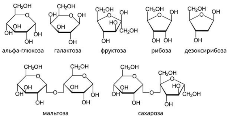
Рис. 6.3. Моносахариды и дисахариды
