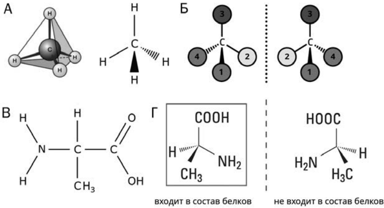
Рис. 4.1. Симметрия и диссимметрия молекул. А – симметричная молекула метана, Б – диссимметрия молекулы, где к углероду присоединены четыре разных радикала, В – демонстрация того, что этим свойством обладают альфа-аминокислоты (кроме глицина), Г – аланин как пример
