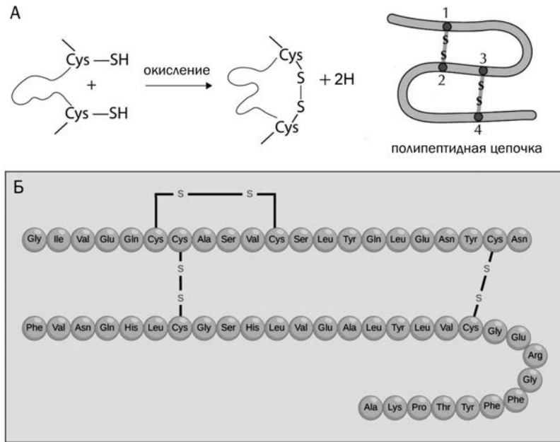
Рис. 3.4. Дисульфидные мостики: общая схема (А) и их место в молекуле инсулина (Б). Обратим внимание, что инсулин состоит из двух независимых полипептидных цепочек, а значит, у него номинально есть четвертичная структура. Заодно мы видим тут и первичную структуру, то есть последовательность аминокислот. N-конец у обеих цепочек находится справа
