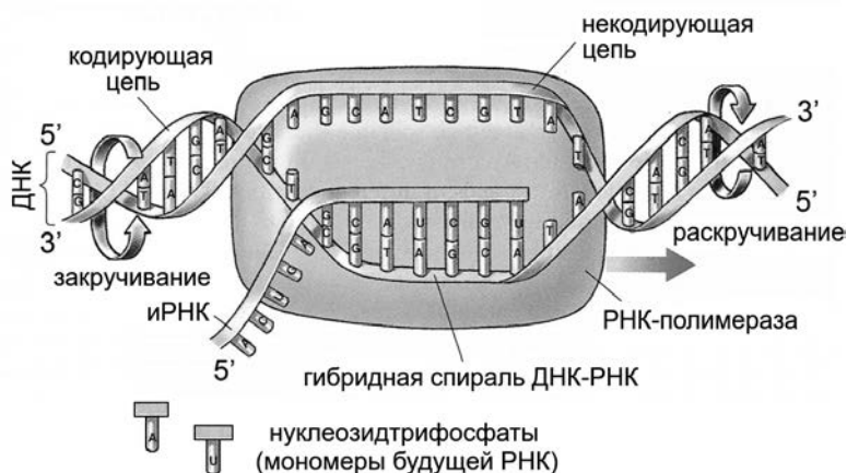
Рис. 9.3. Механизм транскрипции
