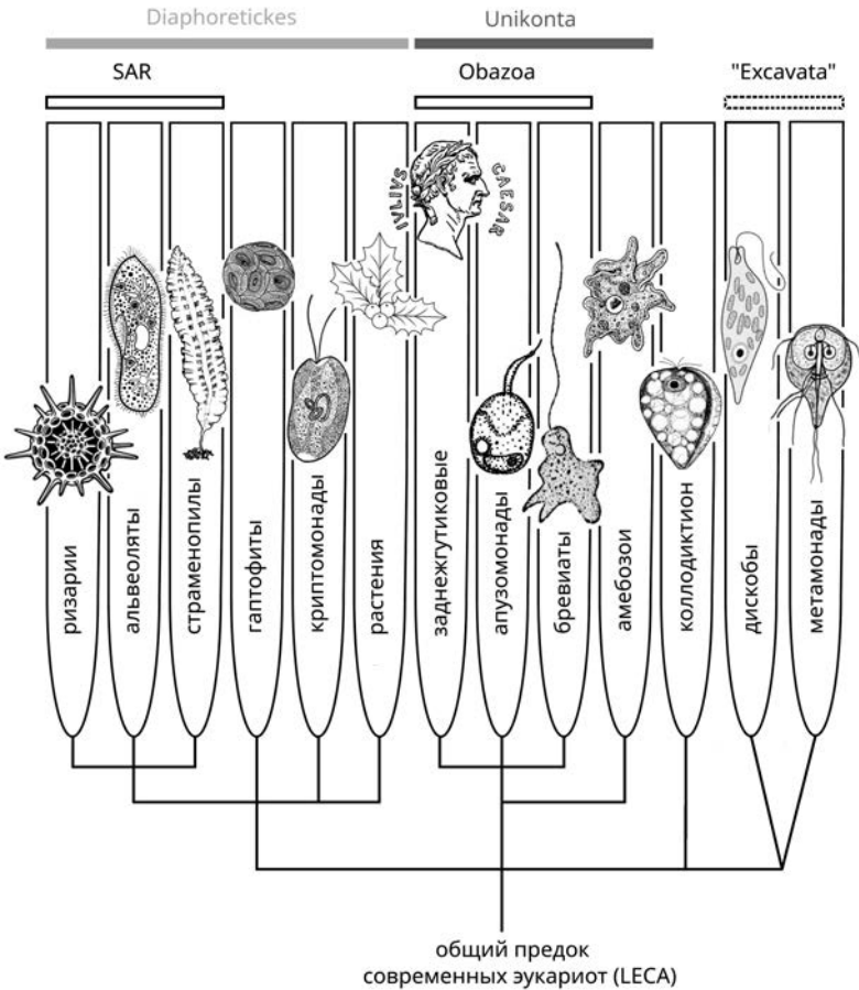
Рис. 15.15. Упрощенное эволюционное древо эукариот, более-менее соответствующее современным представлениям. О положении криптомонад и гаптофит есть целая группа разных гипотез — здесь проблема сознательно оставлена открытой. Проблема родственных связей малых групп внутри Unikonta тоже оставлена открытой, но надо иметь в виду, что сейчас набрала популярность обсуждаемая в тексте гипотеза Obazoa — если она верна, то ветви апузомонад и бревият должны будут примкнуть к опистоконтам. Наконец, далеко не факт, что Excavata действительно являются единой ветвью, а не сборной группой. Подробное обсуждение всех этих нерешенных вопросов — дело будущего, хочется надеяться, что ближайшего, — но уже не этой книги
