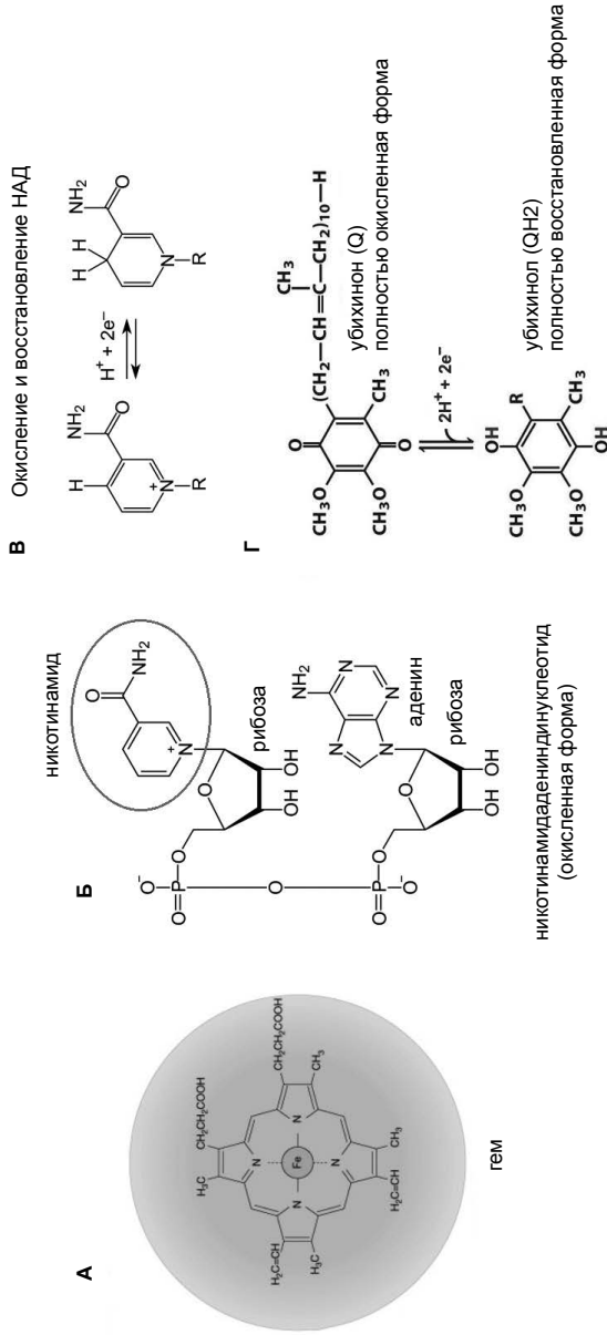
Рис. 11.6. Кофакторы, принимающие участие в процессе дыхания
