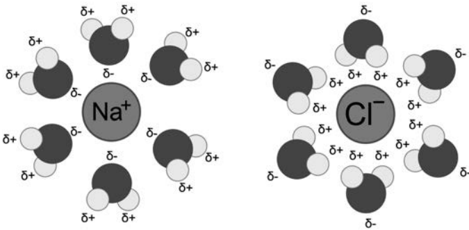
Рис. 2.3. Гидратация ионов
