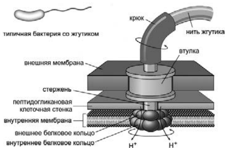
Рис. 11.5. Бактериальный жгутик
