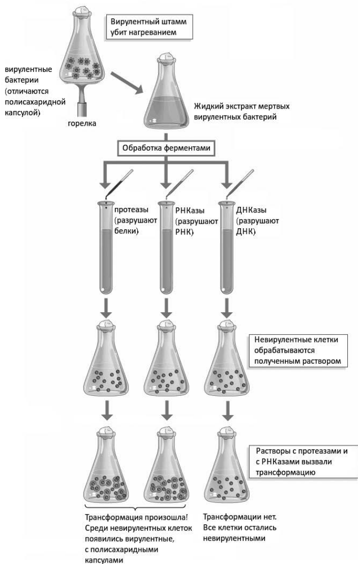
Рис. 8.2. Опыт Эвери
