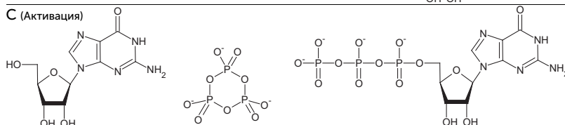
Рис. 10.1. А — последовательность реакций, любая из которых может быть ускорена рибозимом для создания большего числа своих копий. В — синтез нуклеотидов из азотистых оснований и фосфорилированного рибозидного сахара при помощи рибозимов. С — активация нуклеозидов неорганическим триметафосфатом, который образуется из вулканических газов
