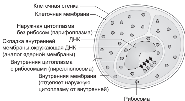
Рис. 18.9. Расположение мембран в клетке бактерий планктомицетов Gemmata obscuriglobis
