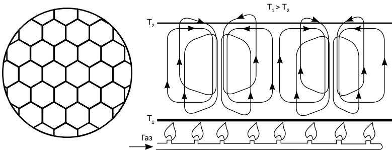
Рис. 5.4. Ячейки Бенара
