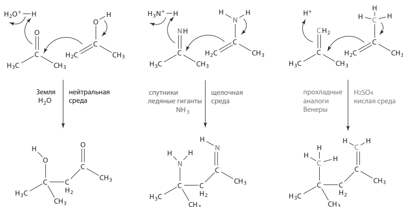
Рис. 12.6. Механизмы формирования связей С-С в разных растворителях. Слева: реакция гликольальдегида с ацетоном в воде проходит благодаря группам C=O (альдольная конденсация, также лежит в основе реакции Бутлераова). В центре: в жидком аммиаке роль C=O могут играть группы C=NH . Справа: в серной кислоте аналогичные реакции идут по связям C=C
