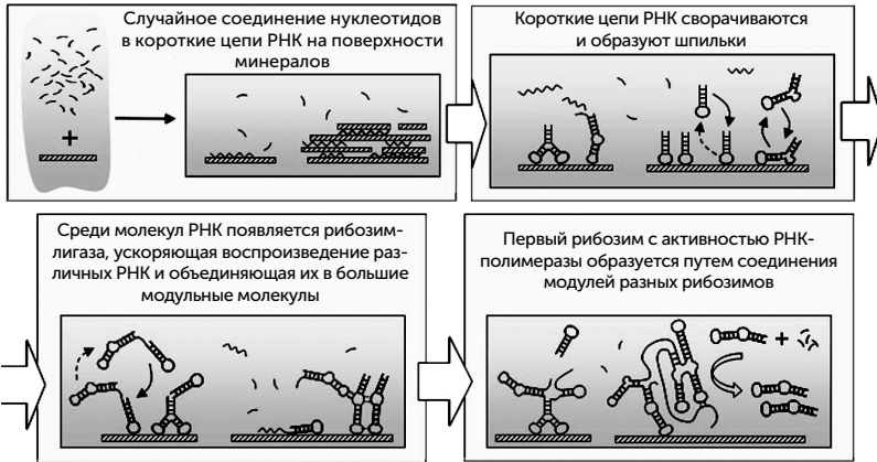
Рис. 9.3. Последовательные стадии эволюции рибозима-полимеразы через сообщество рибозимов-лигаз
