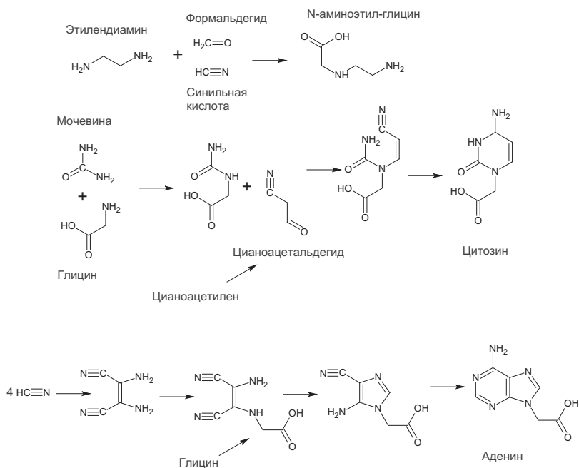
Рис. 12.10. Получение компонентов аминокэтил-глициновой ПНК
