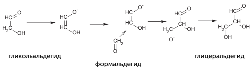
Рис. 10.2. Альдольная реакция (на примере образования глицеральдегида из гликольальдегида и формальдегида)
