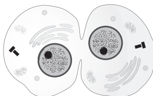
Рис. 18.3. Стадии деления клетки путем митоза
