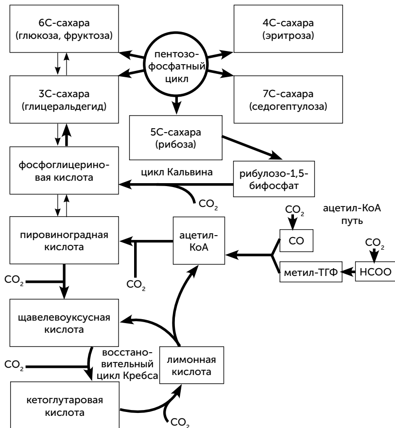
Рис. 11.4. Три основных пути фиксации углекислого газа у различных организмов (цикл Кальвина, ацетил-КоА-путь и восстановительный цикл Кребса) и их связи с остальным обменом веществ. Жирными стрелками показаны реакции, связанные с фиксацией CO 2
