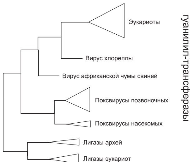
Рис. 18.12. Филогенетическое дерево ферментов пришивания кэпа (гуанилилтрансфераз). Гуанилилтрансферазы происходят от ДНК-лигаз. Ветвь дерева, связывающая ДНК-лигазы с гуанилилтрансферазами, указывает нам на древнейшие гуанилилтрансферазы. Видно, что они принадлежали вирусам, а потом передались эукариотам
