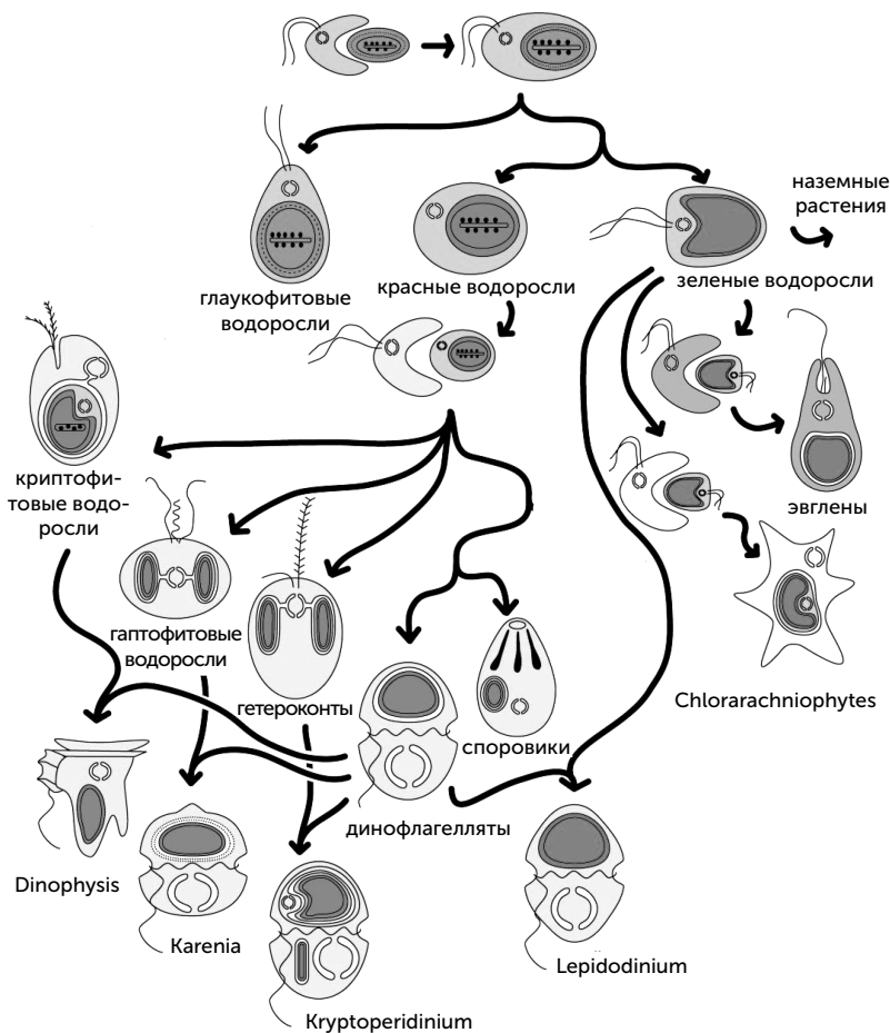
Рис. 18.15. События симбиоза в эволюции различных групп водорослей. Древние эукариоты поселили внутри своих клеток цианобактерии, которые стали хлоропластами. Первые эукариоты с хлоропластами дали начало зеленым, красным и глаукофитовым водорослям. Эвглены и Chlorarachnion произошли благодаря двум эпизодам вторичного симбиоза с зелеными водорослями. Гаптофитовые, криптофитовые, динофлагелляты и гетероконты (группа, включающая бурые, золотистые, желто-зеленые и диатомовые водоросли) произошли путем вторичного симбиоза жгутиконосца с красной водорослью. Динофлагелляты после этого несколько раз теряли хлоропласты и приобретали новые, другого происхождения
