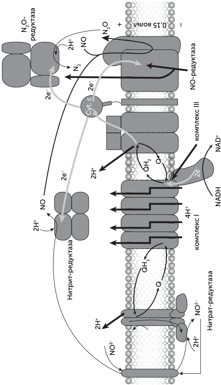
Рис. 17.5. Электрон-транспортная цепь денитрификации. В процессе денитрификации из двух ионов нитрата (NO 3 - ) образуется молекула азота N 2 . На одну молекулу азота по цепи проходит десять электронов. Нитрат-редуктаза Naг превращает нитрат в нитрит (NO 2 - ), используя два электрона с хинона. Нитрит-редуктаза NirS использует один электрон с цитохрома с для восстановления нитрита до оксида азота NO. NO-редуктаза сNог восстанавливает две молекулы NO в одну молекулу закиси азота N 2 O, используются два электрона с цитохрома с. N 2 O-редуктаза Nos превращает N 2 O в азот с затратой двух электронов с цитохрома с.
