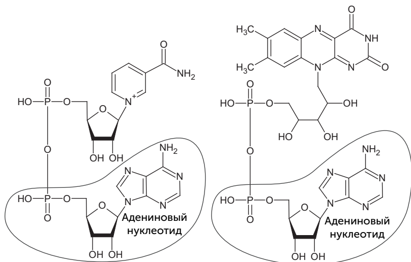
НАД (никотинамид-аденидинуклеотид)
