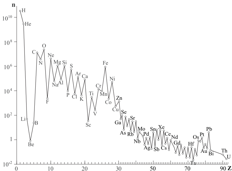
Рис. 12.2. Распространенность элементов во Вселенной
