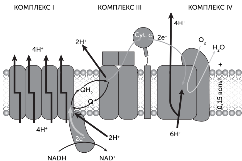
Рис. 15.6. Структура дыхательной цепи аэробного дыхания
