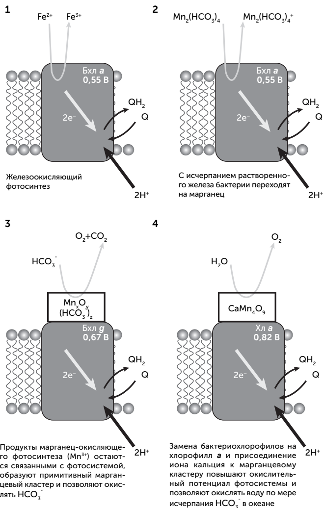
Рис. 16.7. Происхождение кислородного фотосинтеза. По мере истощения запасов растворенного железа ( Fe^{2+} ) предки цианобактерий перешли на окисление марганца ( Mn^{2+} ). Из окисленных атомов марганца ( Mn^{3+} ) собрался примитивный марганец-кислородный кластер, который позволил клеткам окислять бикарбонат ( HCO_3^- ) с выделением кислорода и CO_2 . Дальнейшее совершенствование этой системы включало замену бактериохлорофиллов на хлорофилл а (более сильный окислитель) и добавление кальция к марганец-кислородному кластеру, что позволило окислять не только бикарбонат, но и воду
