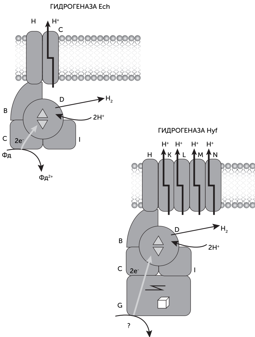
Рис. 17.8. Строение комплекса I и родственных ферментов. Латинскими буквами обозначены субъединицы комплекса I и их гомологи в других ферментах. Цитоплазматические субъединицы принимают электроны от внешних источников (ферредоксин, муравьиная кислота, НАДН) и передают на гидрогеназную субъединицу D, выделяющую водород. В комплексе I гидрогеназный центр субъединицы D неактивен, и электроны передаются дальше на хинон. Мембранные субъединицы K, L, M и N переносят протоны через мембрану. Количество перенесенных протонов определяется количеством этих субъединиц в составе комплекса. Гидрогеназа Ech переносит один протон на пару прошедших электронов, гидрогеназа Huf и комплекс I — четыре
