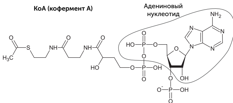
Рис. 10.3. Строение различных коферментов: НАД (слева сверху), ФАД (справа сверху), КоА (снизу). Адениновый нуклеотид обведен
