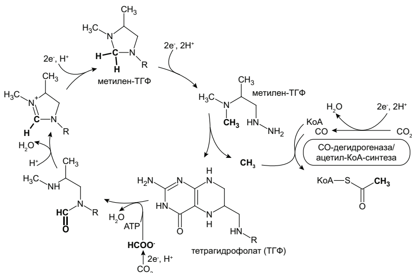
Рис. 11.3. Восстановительный ацетил-КоА-путь фиксации CO 2 . Жирным шрифтом выделен атом углерода, проходящий восстановление на тетрагидрофолате
