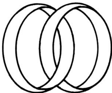
Рис. 27. Простейшее зацепление — символ бракосочетания
