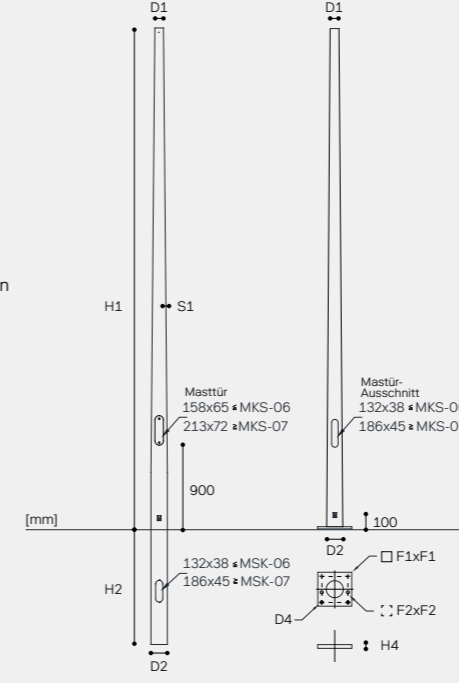
MKS (-F) Aufgesetzte Masttür
