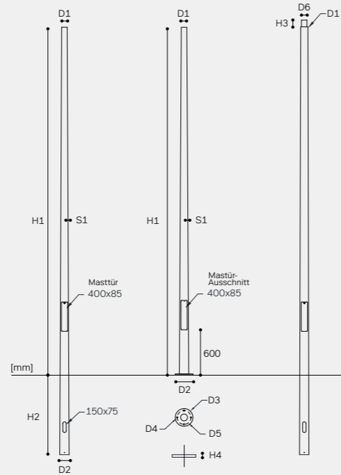
MKG (-F) / M-DFC Flächenbündige Masttür
