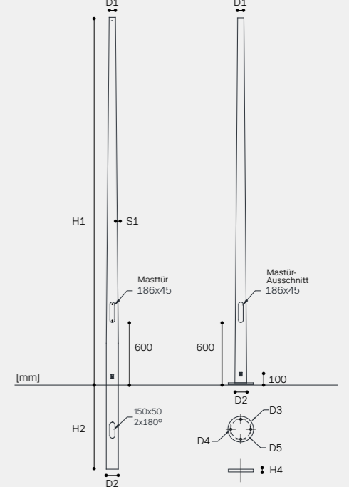
MKI (-F) Masttür „RESET“
