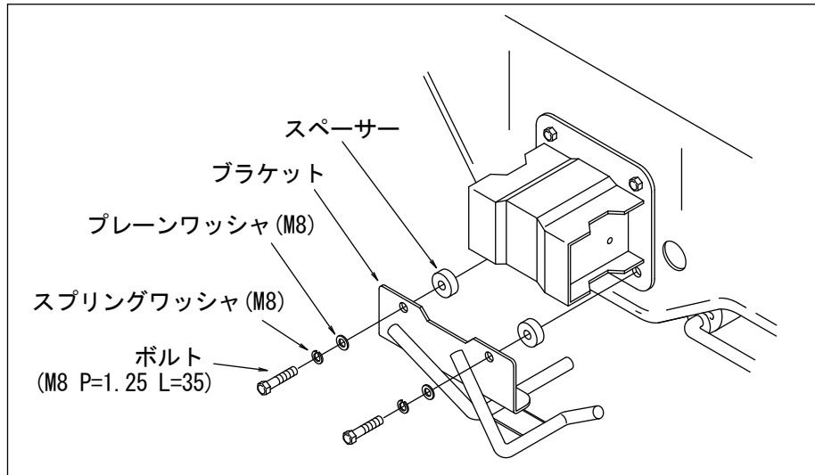
【 図3. ブラケット取付け図 】
