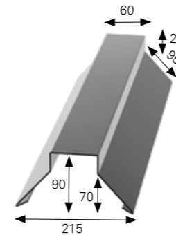
TRAPÉZ GERINCLEMEZ
