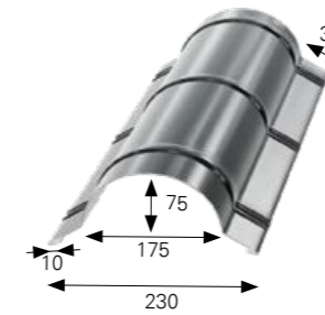
FÉLKÖRÍVES GERINCLEMEZ
