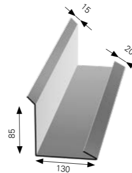
FALSZEGÉLY II
