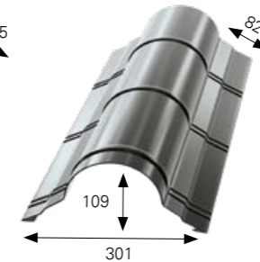
FÉLKÖRÍVES GERINCLEMEZ SZÉLES
