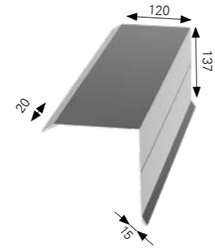
OROMDESZKA SZEGÉLY I
