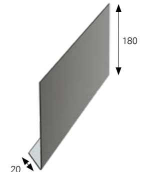
ALSÓ ERESZSZEGÉLY
