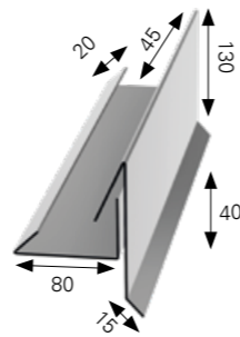
OROMDESZKA SZEGÉLY II
