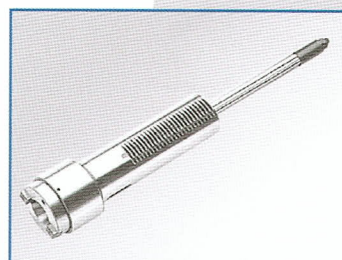
CODE 40020: Achse Spindel ISO 40 + Zugstange (DIN 2080) Axe broche ISO 40 avec tirant (DIN 2080)
