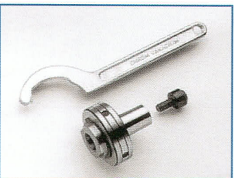
CODE 39000050/60/70: Kegel mit Sicherungsringmutter für Schafffräser, mit Innenklemmen auf Anfrage 1-2-3 Cône avec écrou de serrage pour fraises à queue conique, avec morse interne sur demande 1-2-3
