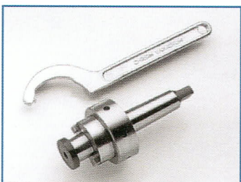
CODE 39000010/20/30/40: Kegel mit Sicherungsringmutter für Planfräser, mit Anschluss auf Anfrage ø 16-22-27-32. Cône avec écrou de serrage pour fraises à surfacer, avec raccord sur demande ø 16-22-27-32.
