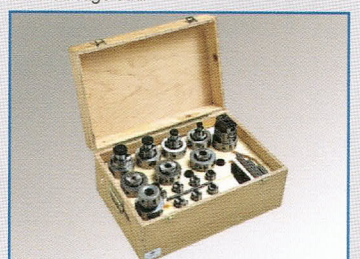
CODE 9459210 (CM4) CODE 9459212 (ISO 40): Kasten komplett mit Kegel für Schafffräser, Planfräser, Zangenträgerspindel ø 4-20, Stäberkopf ø 70 mit Anschluss CM4, auf Anfrage Anschluss ISO 40. Coffret incluant cônes pour fraises à queue conique, pour fraises à surfacer, mandrin porte-pinces ø 4-20, tête aléseuse ø 70 avec raccord CM4 sur demande raccord ISO 40.
