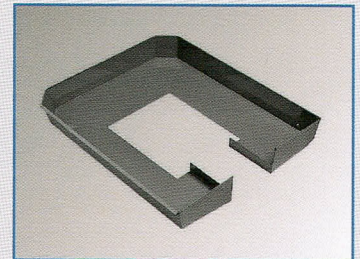
CODE 5355351: Späneauffangbehälter für TCS Cuvette de récupération des copeaux pour TCS
