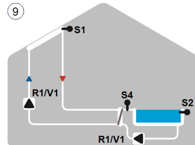
9 Solar mit Wärmetauscher und Pool 1
