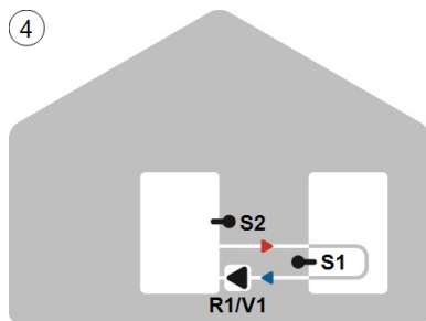
4 Speicherumladung
