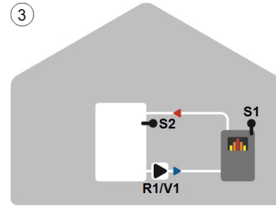
3 Feststoffkessel mit Speicher
