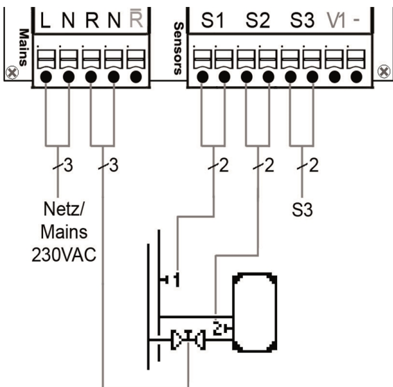
Programm 8 Sperrventil
