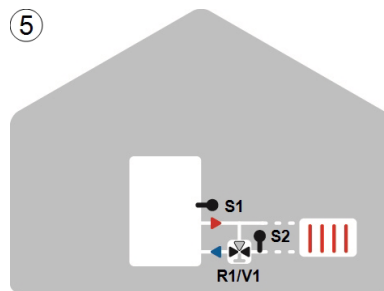
5 Heizkreis-Rücklaufanhebung
