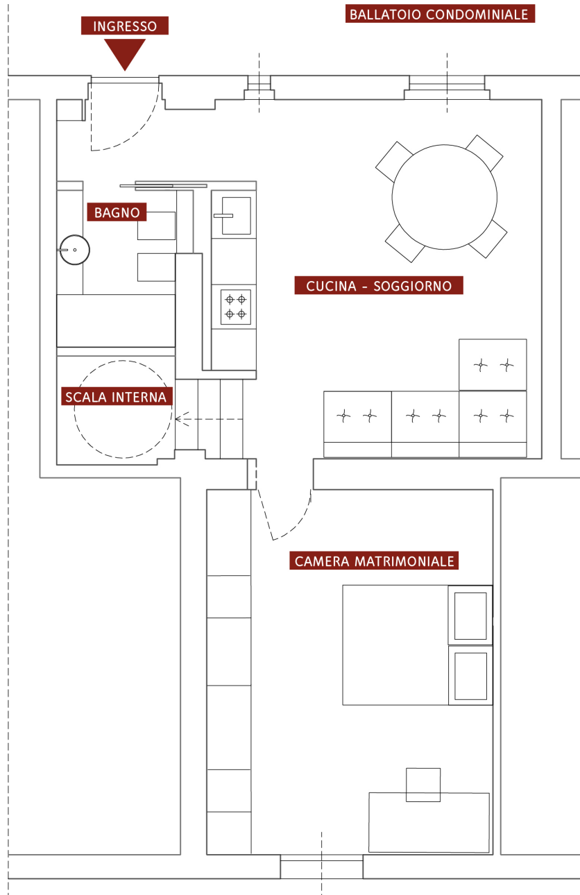
PIANTA PIANO 4°
