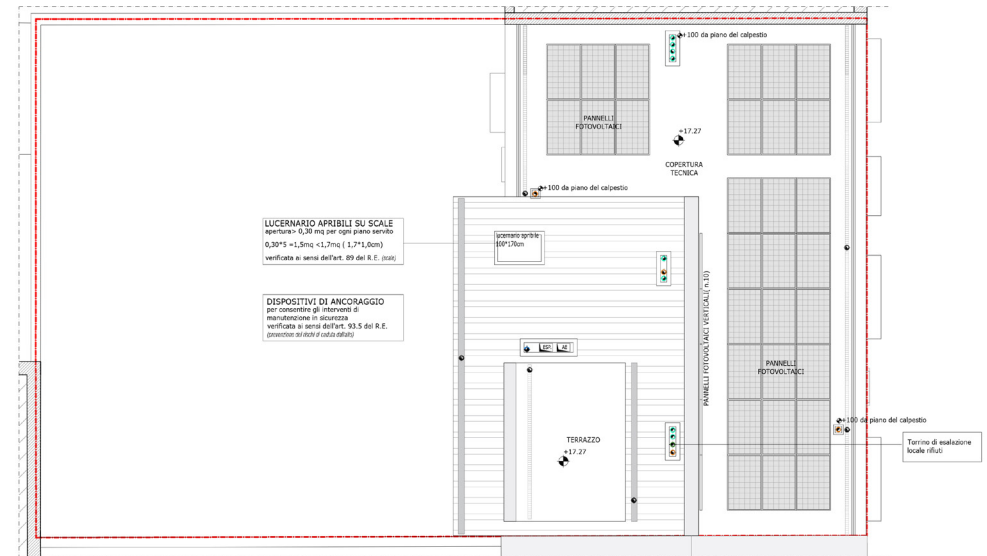
PIANTA PIANO COPERTURA
