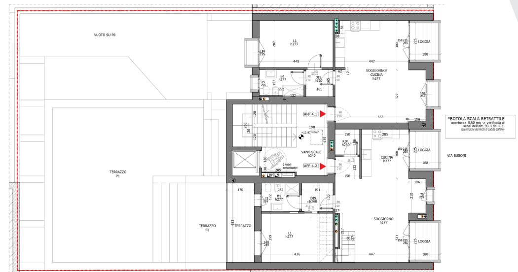
PIANTA PIANO QUARTO
