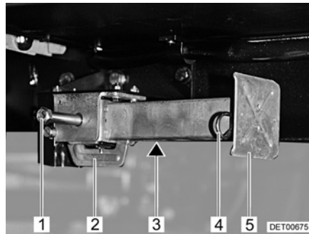
Kuva 15 Nostotuki
