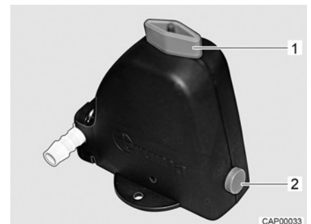
Kuva 106 Varmuus-/vedenpoistiventtiili auki
