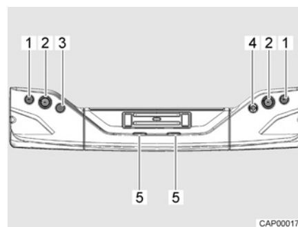
Kuva 125 Valaistus takaosa
