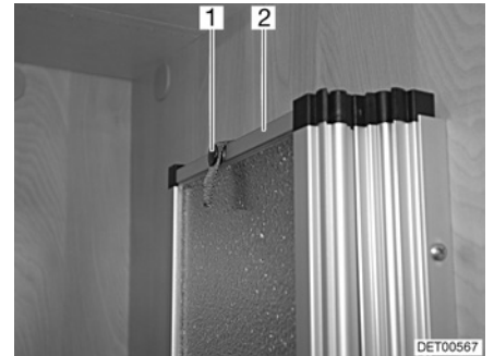
Kuva 113 Kiinnitys, suihkuseinä
