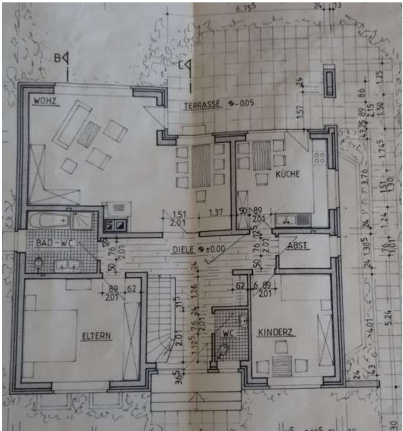
Bauplan EG
