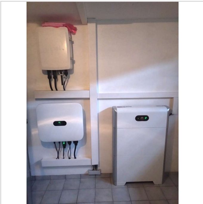
Wechselrichter-Batteriespeiche
