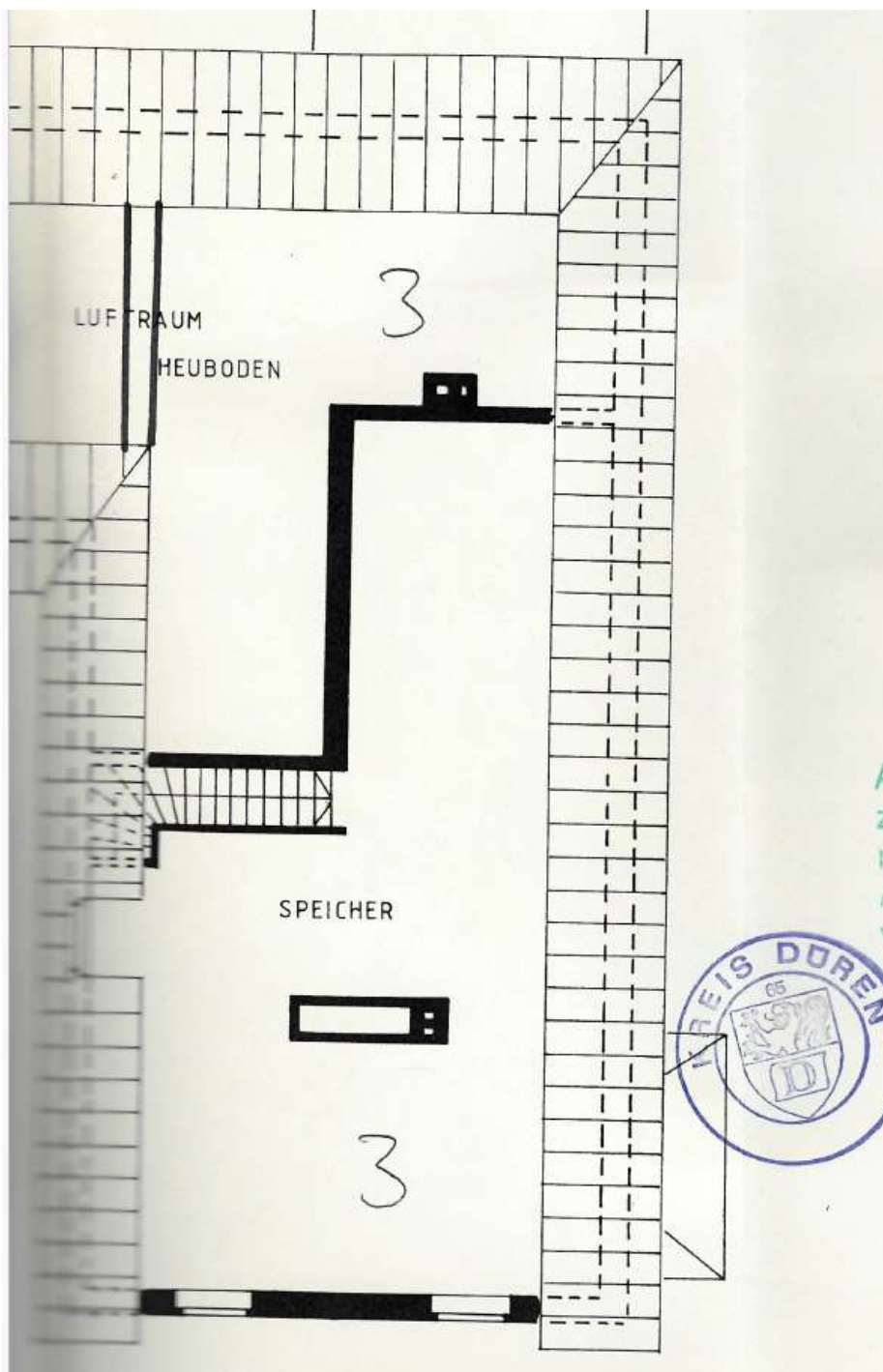
Speicher Haupthaus
