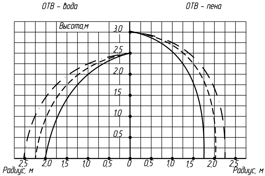
Ороситель эвольвентный "ОЭ-16" (Р от 0,15 до 0,30МПа включительно)
