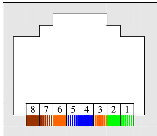
Рис. 3. Нумерация контактов
