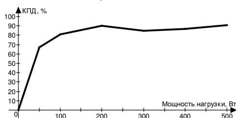
Рисунок 4.1. График зависимости КПД усилителя МРА-21хх от мощности нагрузки 1 .
