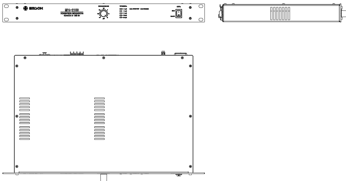
Рисунок 7.1. Расположение вентиляционных отверстий.
