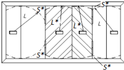
Рисунок 5. Защита немонолитной конструкции. ( S^* < 0,1 м^2 , L < L^* )
