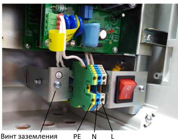
Рисунок 3.5.1 – Узел подключения питания.
