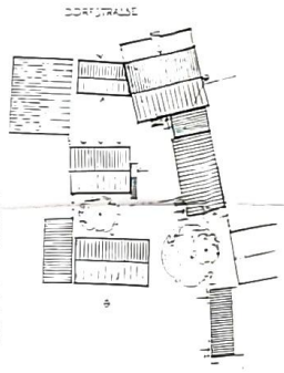
LAGEPLAN 1:1000
