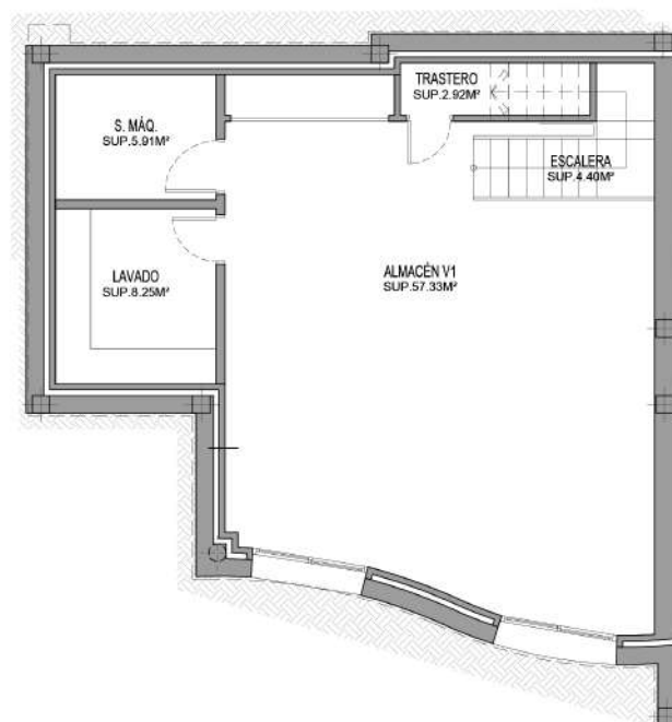
Planta Sótano
