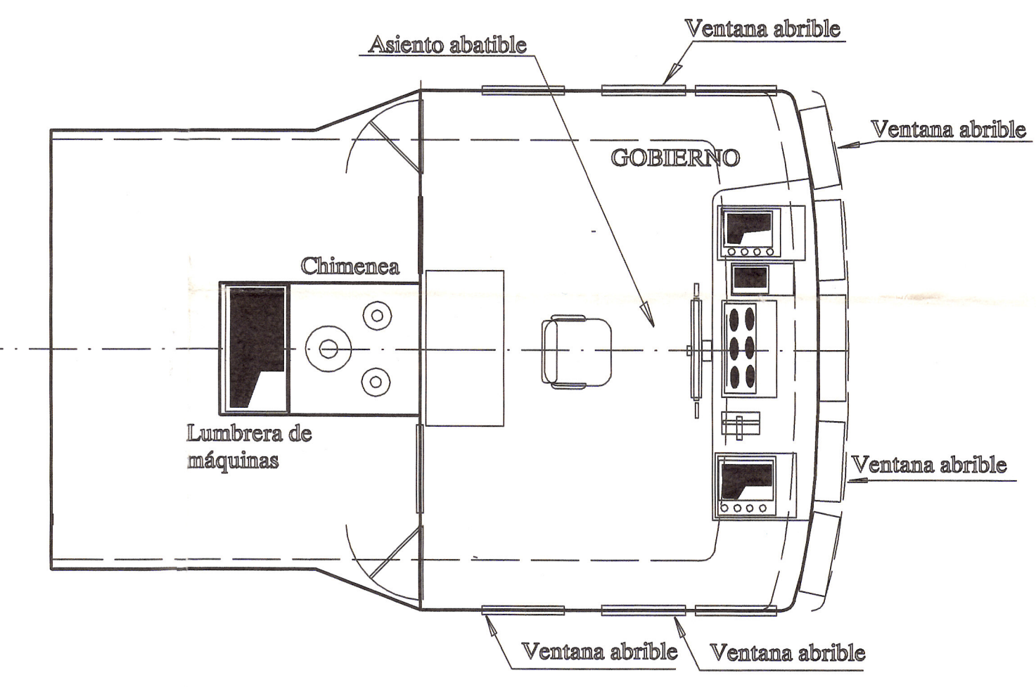
CUBIERTA PUENTE
