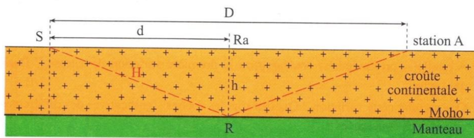
Figure 4.25 - Document 1 : Propagation des ondes P réfléchies (ondes PMP) dans la croûte terrestre
