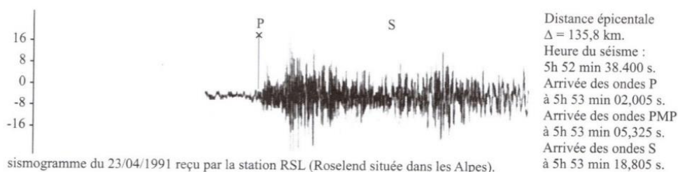
Figure 4.25 - Document 1 : Propagation des ondes P réfléchies (ondes PMP) dans la croûte terrestre
