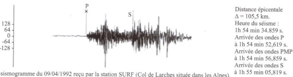
Figure 4.26 - Sismogrammes à étudier
