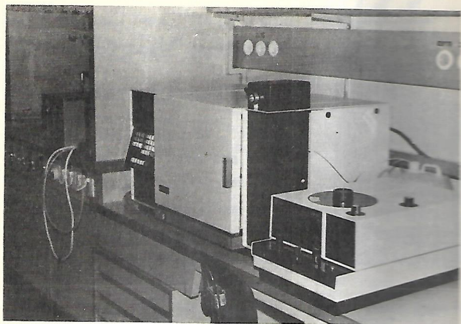
המכשיר לכרומטוגרפיה נוזלית בלחץ גבוה (HIGH PRESSURE LIQUID CHROMATOGRAPHY)
