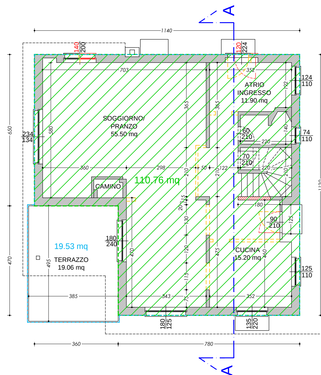
PIANTA PIANO TERRENO
