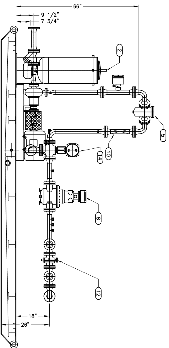
ELEVATION
