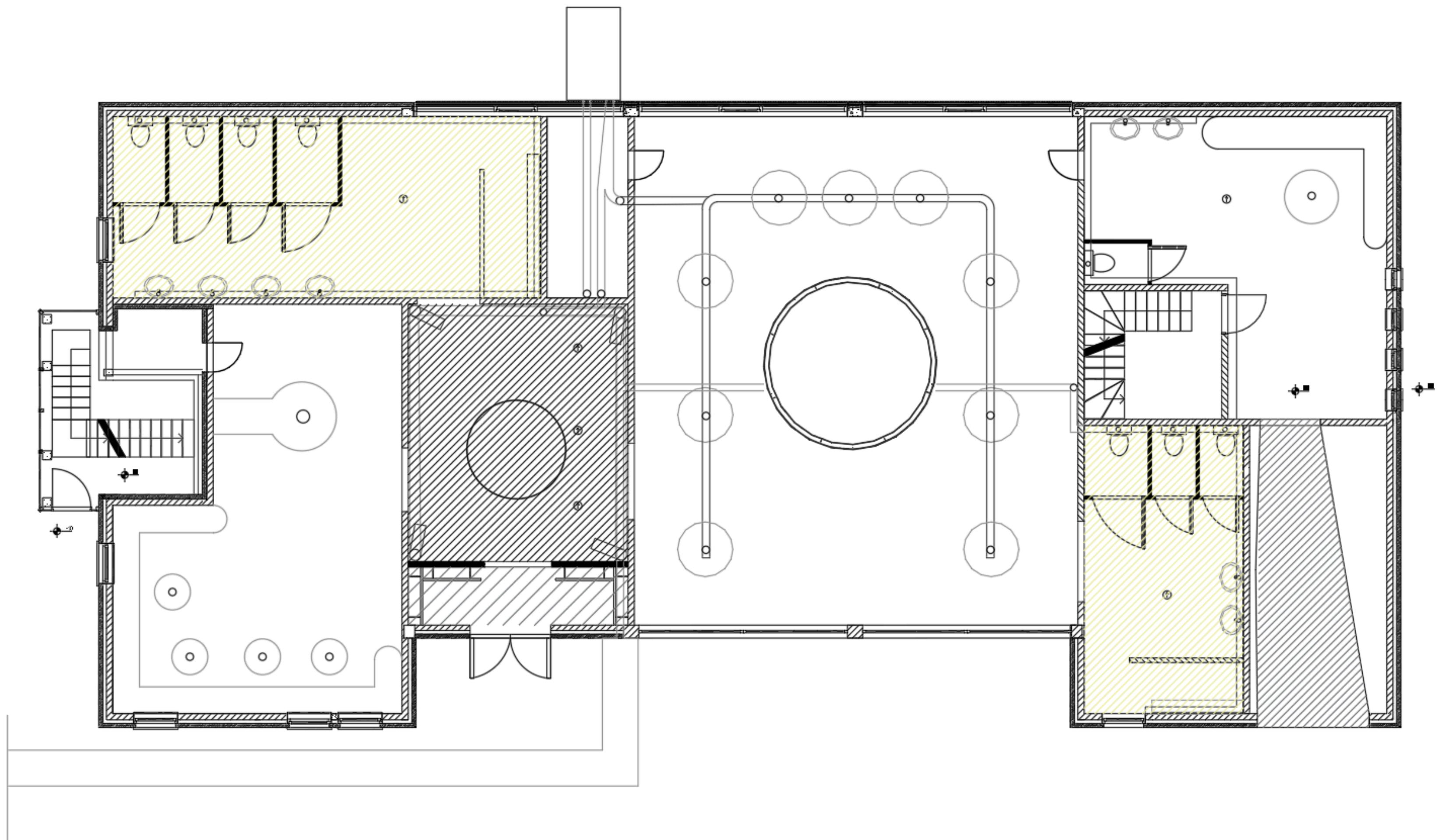
GRONDPLAN: aanduiding kleuren lichtzones
