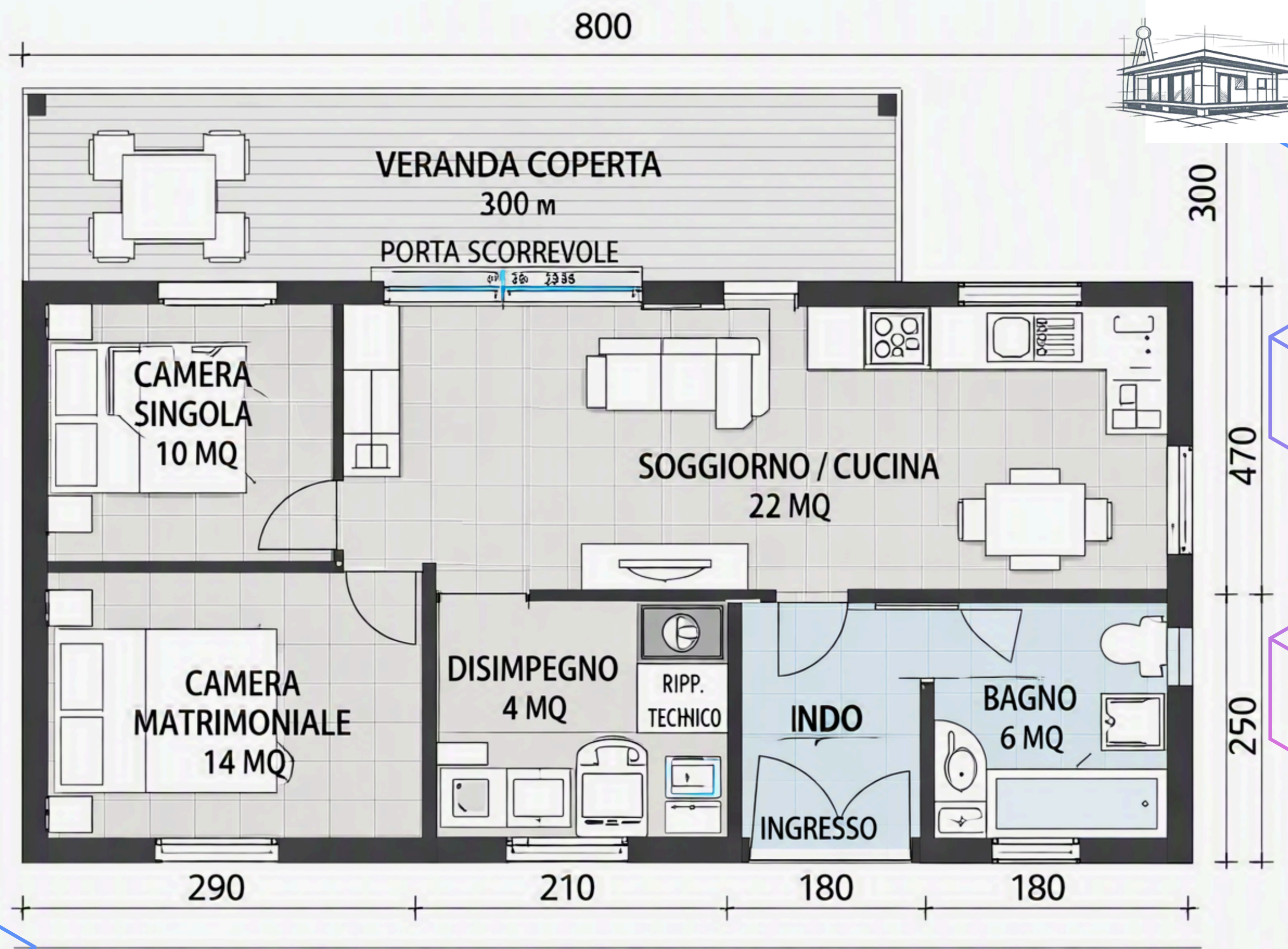
PIANTA CASA MODULARE – 60 MQ
