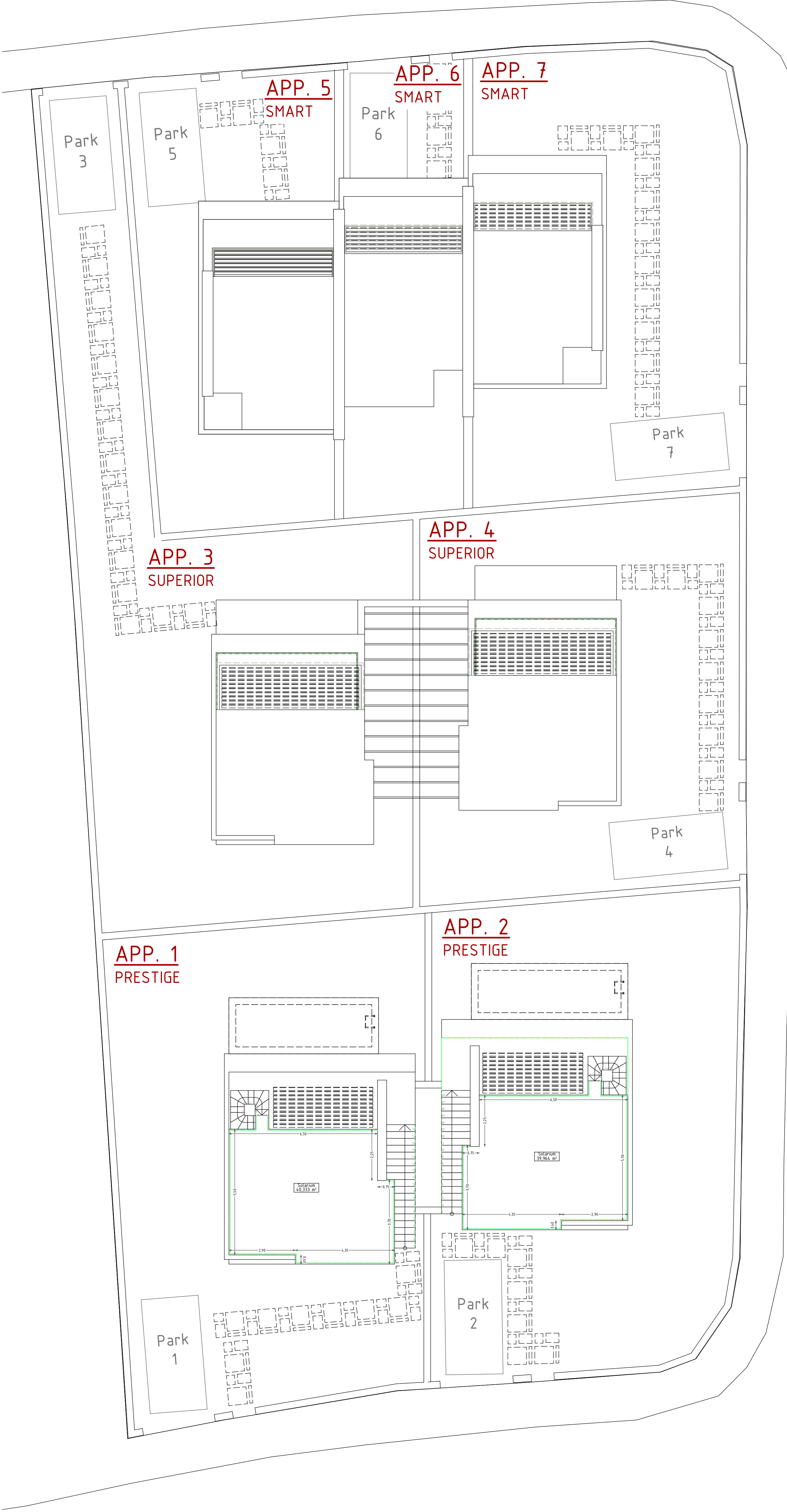
PIANTA PIANO COPERTURA
